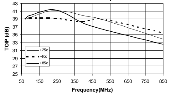
TOIP vs Temp
