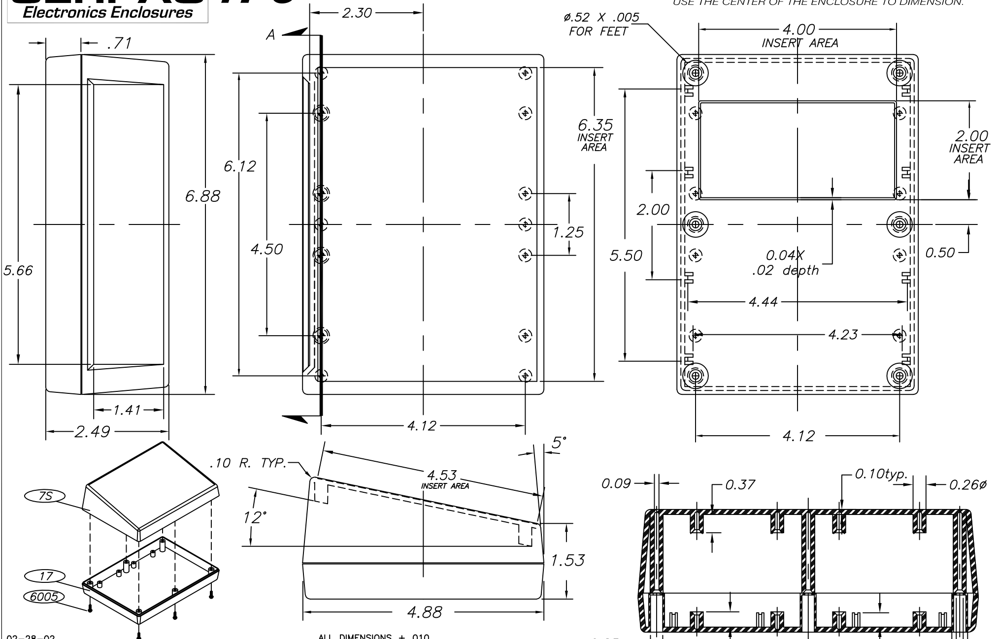
SECTION A-A
